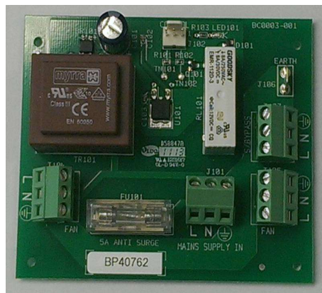
BP40762 'MB' & 'HMB' Power PCB
